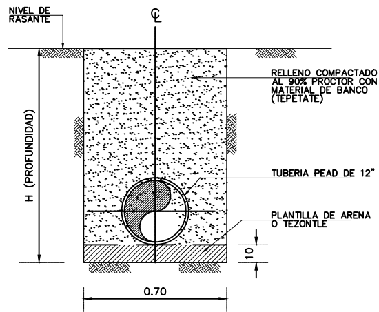
SECCION CONSTRUCTIVA DE ZANJA
