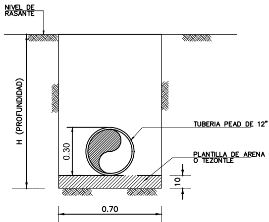
EXCAVACION DE ZANJA
